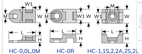
HC-0,0L,0M HC-0R HC-1,1S,2,2A,2S,2L
