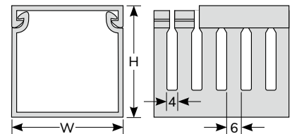
HVD SLOT : 4mm
