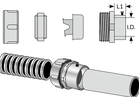
(Metal flexible conduit) EBG (EMT pipe)
